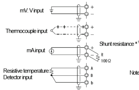
Input wiring
